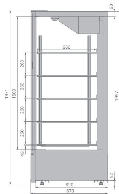
SHKAFF 0,7/1,4 HT
