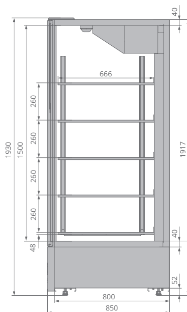
SHKAFF 0,7/1,4 CT
